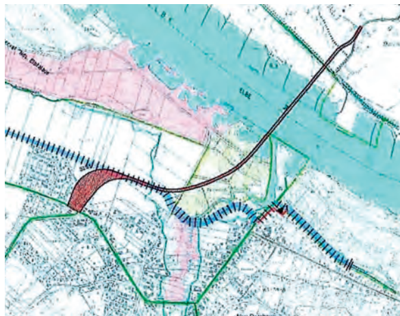
Die harmonisierte Vorzugstrasse für die Elbbrücke mit Ortsumfahrung von Neu Darchau ist rot gekennzeichnet, die informativ zur Erläuterung ergänzte mögliche Linie einer Hochwasserschutzanlage violett.
